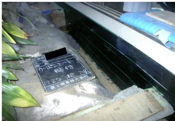
炭素繊維シート貼付状況
